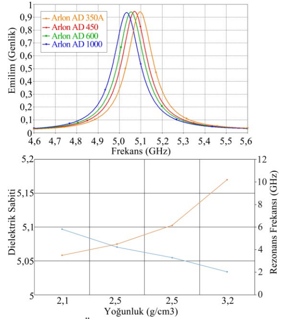
Şekil 5. (a) Önerilen yapıya arlon malzeme eklenerek oluşturulan yoğunluk sensör grafiği ve (b) arlon yoğunluğunun dielektrik sabiti ve rezonans frekansına bağlı değişimi
