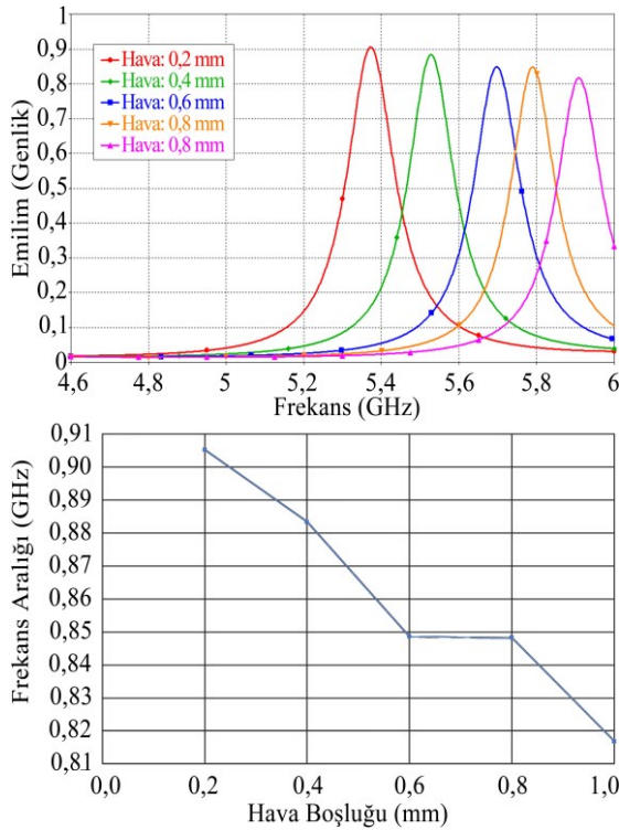
Şekil 4. (a) Önerilen yapıya hava katmanı eklenerek oluşturulan basınç sensör grafiği ve (b) hava katman kalınlığının frekansa bağlı değişimi
