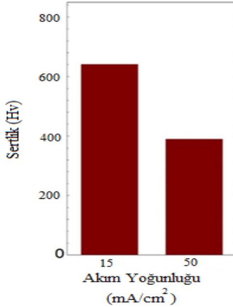
Şekil 4. Ni-B alaşım kaplamaların mikrosertliği üzerinde akım yoğunluğunun etkisi (TMAB banyo kons. 3 g/l)
