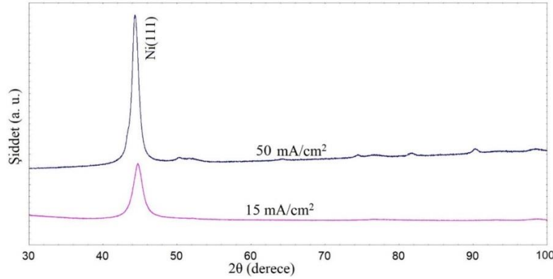
Şekil 3. Ni-B alaşımı kristal yapısına akım yoğunluğunun etkisi (TMAB banyo konsantrasyonu 3 \text{ g/l} ).
