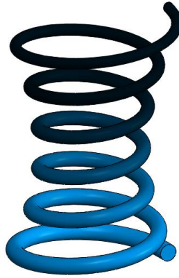
Şekil 2. Fonksiyonel derecelenmiş malzemeli değişken kesitli hiperbol helis
